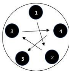
5 Lug Tightening
