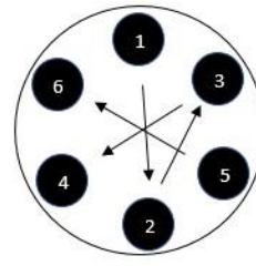
6 Lug Tightening
